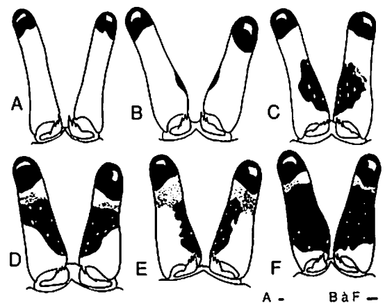
FIG. 8. — Variation de la pigmentation sur les pédoncules oculaires de Calcinus vachoni (échelles 1 mm) : A-E, MNHN Pg5501 ; F, MNHN Pg5503. A, ♂ 2,9 mm ; B, ♂ 2,2 mm ; C, ♂ 2,2 mm ; D, ♀ 1,9 mm ; E, ♂ 1,9 mm ; F, ♂ 2,1 mm.
