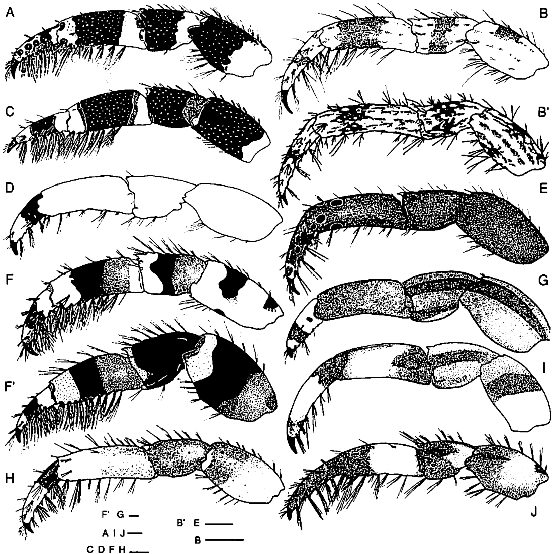
FIG. 3. — Calcinus avec des taches ou bandes colorées sur le troisième périopode (dessin du périopode gauche ; échelles 1 mm). A, C. elegans , ♂ 7.5 mm, Mangareva (Pg5383) ; B, C. gauti , ♀ ov. 2.6 mm holotype, Moruroa (Pg5412) ; B', C. pulcher , ♂ 3.5 mm, île Cocos (WAM 561-89, redessiné d'après Morgan 1991, fig. 45) ; C, C. orchidae , ♂ 4.5 mm holotype, Nuku Hiva (Pg5469) ; D, C. guamensis , ♀ 4.2 mm, Hiva Oa (Pg5391) ; E, C. haigae , ♂ 4.2 mm, Moruroa (Pg5392) ; F, C. isabellae , ♂ 4.6 mm holotype (Pg5470) ; F', C. imperialis , ♂ 11.0 mm, Nouvelle-Calédonie (Pg3428) ; G, C. laevimanus , ♂ 10.2 mm, Moruroa (Pg5467) ; H, C. latens ♂ 5.6 mm, Moruroa (Pg5408) ; I, C. seurati , ♂ 5.3 mm, Tahiti (Pg5414) ; J, C. spicatus , ♂ 6.3 mm, Moruroa (Pg5418).
