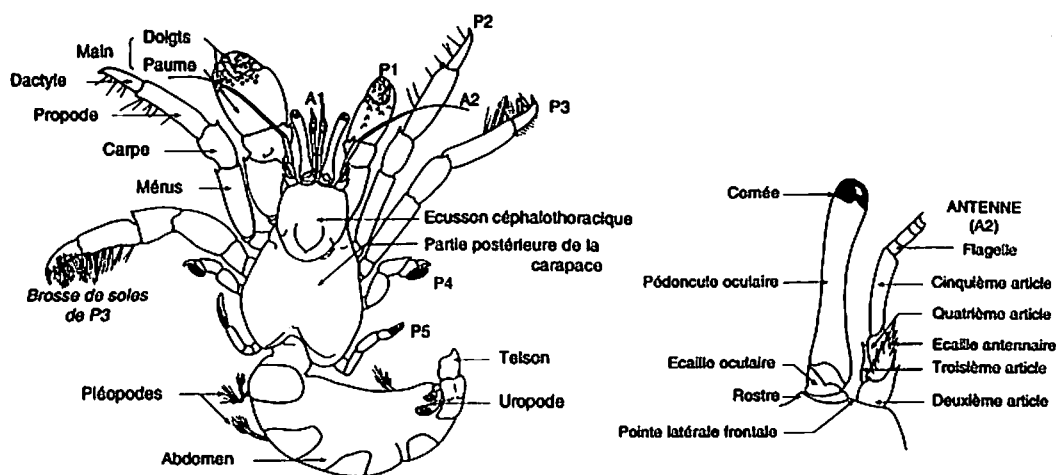
FIG. 1. — Définition des termes utilisés : A1 et A2, antennules et antennes ; P1, premier péréiopode ou chélicède ; P2 et P3, deuxième et troisième péréiopodes ou pattes ambulateurs ; P4 et P5, quatrième et cinquième péréiopodes.
