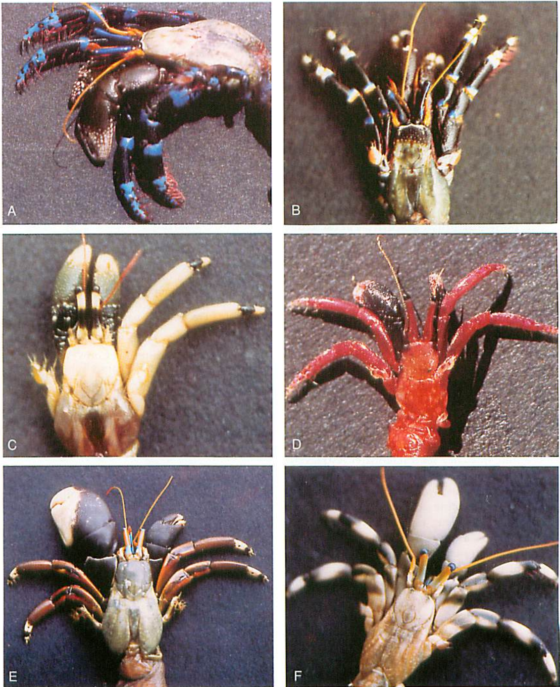
FIG. 4. — Coloration des Calcinus . A, C. elegans , ♂ 7,5 mm, Mangareva (Pg5383) ; B, C. orchidae , ♂ 4,5 mm holotype, Nuku Hiva (Pg5469) ; C, C. guamensis , ♀ 4,2 mm, Hiva Oa (Pg5391) ; D, C. haigae , ♂ 2,3 mm, Moruroa (Pg5392) ; E, C. laevimanus , ♂ 10,2 mm, Moruroa (Pg5467) ; F, C. seurati , ♂ 5,0 mm, Moruroa (Pg5415).
