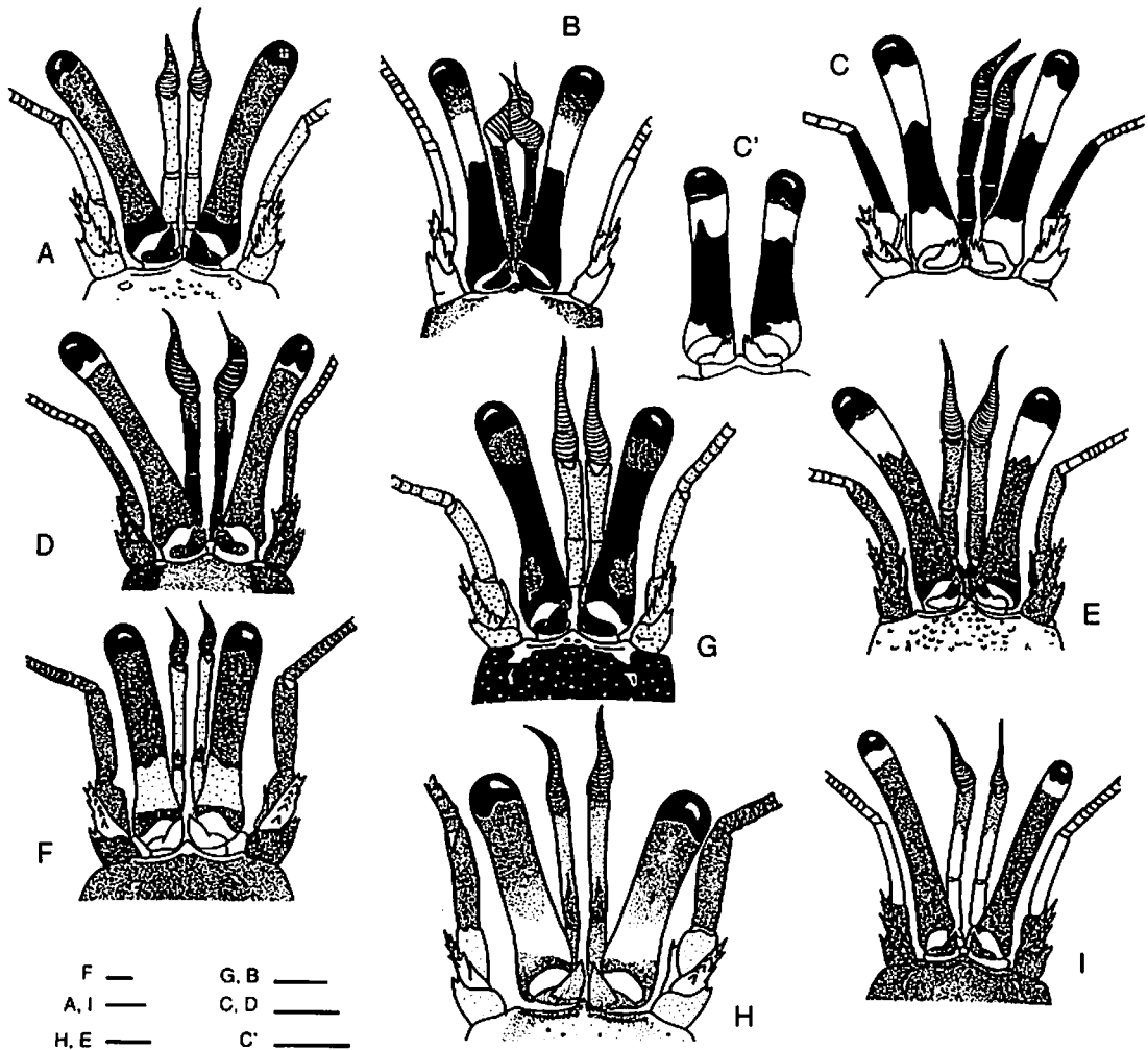
FIG. 2. — Calcinus avec des bandes colorées sur les pédoncles oculaires. A, C. elegans , ♂ 7.5 mm, Mangareva (Pg5383) ; B, C. gaimardii s.l., ♂ 4.3 mm, Tahiti (Pg5387) ; C, C. guamensis , ♀ 4.2 mm, Hiva Oa (Pg5391) ; C', Id. , ♀ ov. 2.9 mm, Hiva Oa (Pg5390) ; D, C. haigae , ♂ 4.2 mm, Moruroa (Pg5392) ; E, C. isabellae , ♂ 4.6 mm holotype (Pg5470) ; F, C. laevimanus , ♂ 10.2 mm, Moruroa (Pg5467) ; G, C. orchidae , ♂ 4.5 mm holotype, Nuku Hiva (Pg5469) ; H, C. seuratii , ♂ 5.3 mm, Tahiti (Pg5414) ; I, C. spicatus , ♂ 6.3 mm, Moruroa (Pg5418). Échelles 1 mm.
